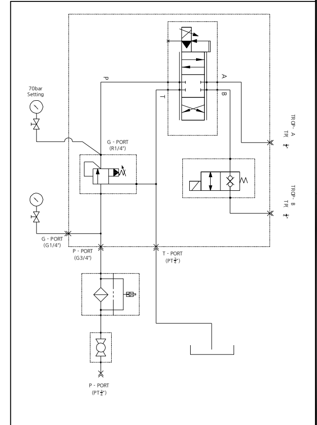
HYD. DIAGRAM
